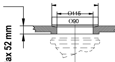
Max 52 mm ÄRAVOOLU AVA
