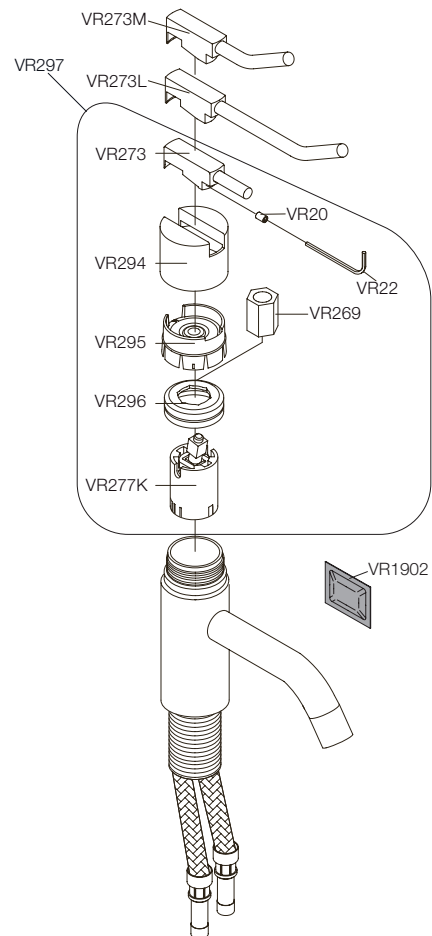
Ventiil ja käepide alates 2011
