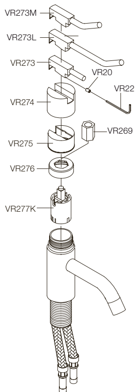
Ventiil ja käepide enne 2011
