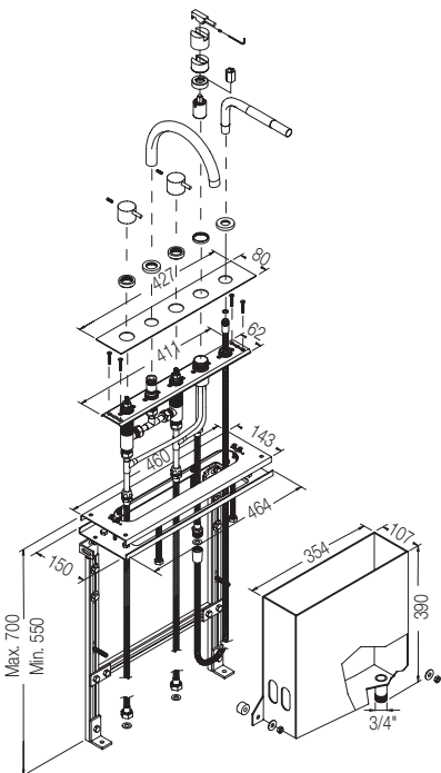
Komplektis paigaldusraam ja vee kogumise nõu (BK System)
