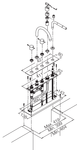
Ilma paigaldusraami ja vee kogumise nõuta (BKA System).
